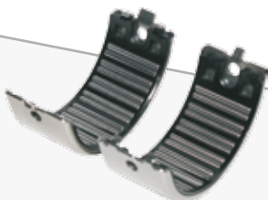
Jogo de Rolamento P/ Freio à Disco Pneumático (Ø65,4X27,80 mm) I Pareja de Alojamientos y Rodamientos del Balancín (Ø65,4X27,80 mm) I Caliper Roller Bearing Set (Ø65,4X27,80 mm)
