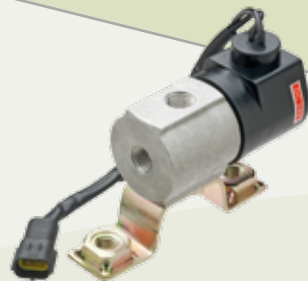
Cj Válvula Solenóide 3 / 2 Vias 24 V (VW) | Válvula Solenóide 3 / 2 Vias (24 V) | Solenoid Valve (24 V) N.º FARJ: 47275-273 CONV. P: 2RP901015 (VW) / 2T0907631 (VW) / 2TJ901015 (VW) APLIC.: VW: 13.170E / 15.170E / 15.190E / 17.250E / 19.320E / 23.250E / 24.250E / 26.260E / 31.260
